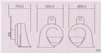
FANFARE TYPE
